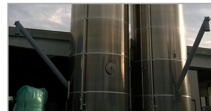
COCLEE TUBOLARI ESTRATTRICI DA SILOS TUBULAR DISCHARGE SCREWS FROM SILOS
