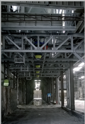
SILOS SU STRUTTURA CON SCARICATORE TELESCOPICO PER CARICO AUTOBOTTE SILOS WITH DISCHARGE SCREW FOR LOADING TANK TRUCKS
